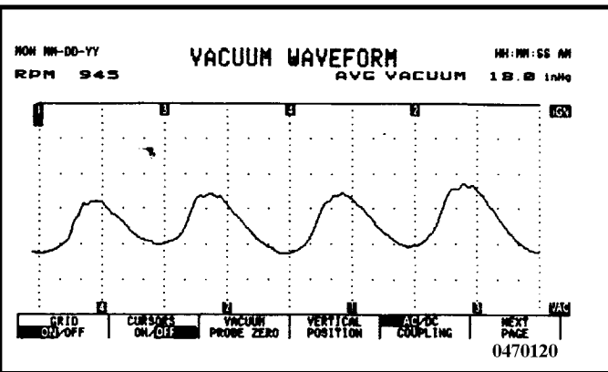
四缸引擎正常波形
