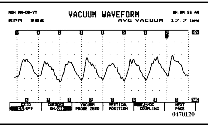
八缸引擎正常波形
