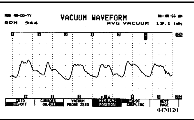
六缸引擎正常波形
