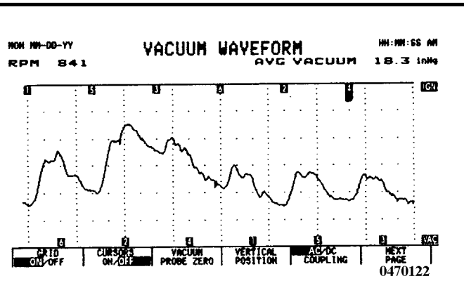
第四缸排氣門間隙太大
