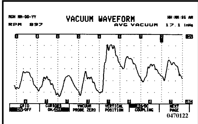
第一缸排氣門彈簧斷裂
