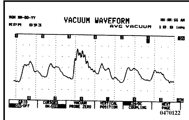
第二缸活塞環缺口再同一直線
