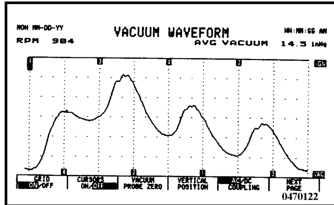
第四缸排氣門面燒毀
