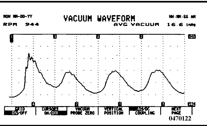
第四缸排氣門搖臂斷裂
